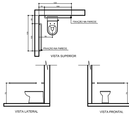
DET. 02 (I.S. ESPECIAL) ESC. 1:25
