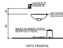
DET. 03 (PIA PADRÃO) ESC. 1:25
