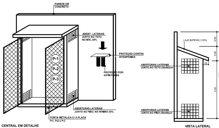
DET. 02 (I.S. ESPECIAL) ESC. 1:25
