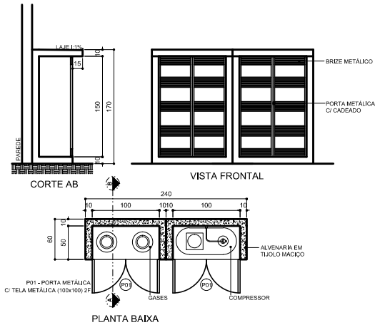
DET. 04 (COMPRESSOR e GASES MEDICINAIS) ESC. 1:25
